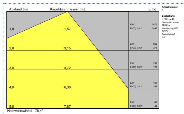
Kegeldiagramm
