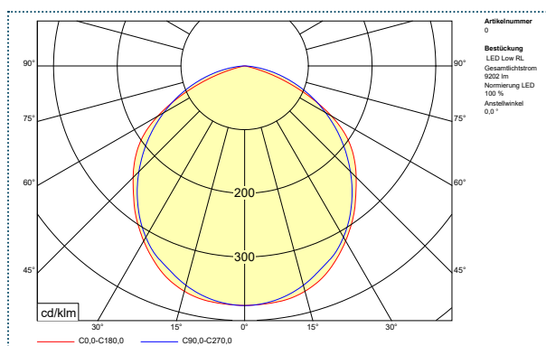
Lichtstärkeverteilung / polar
